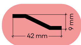
Perfil / Section
